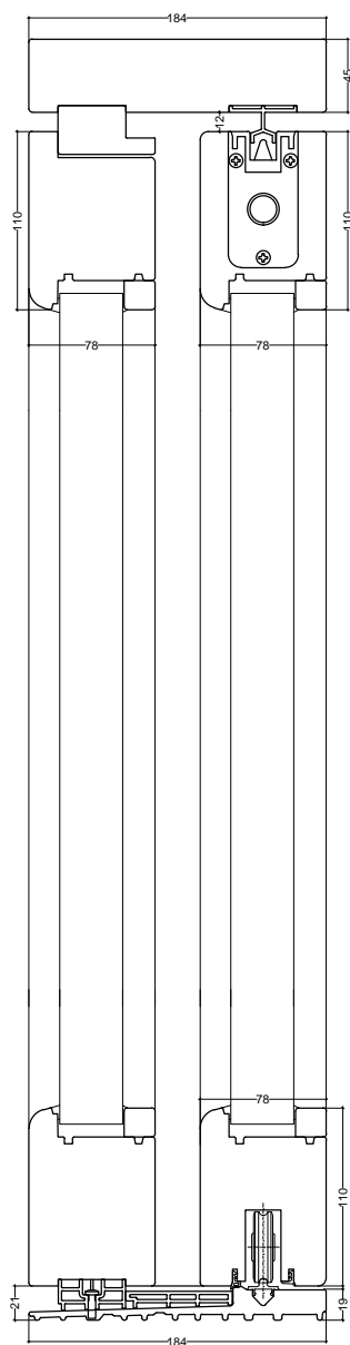
Sezione orizzontale
