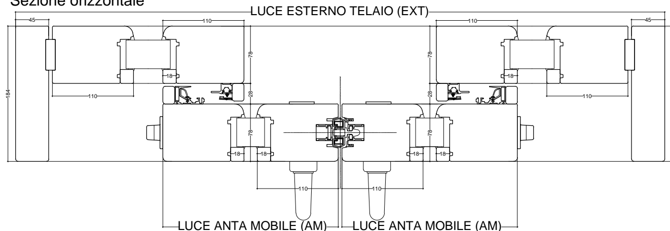
Sezione orizzontale
