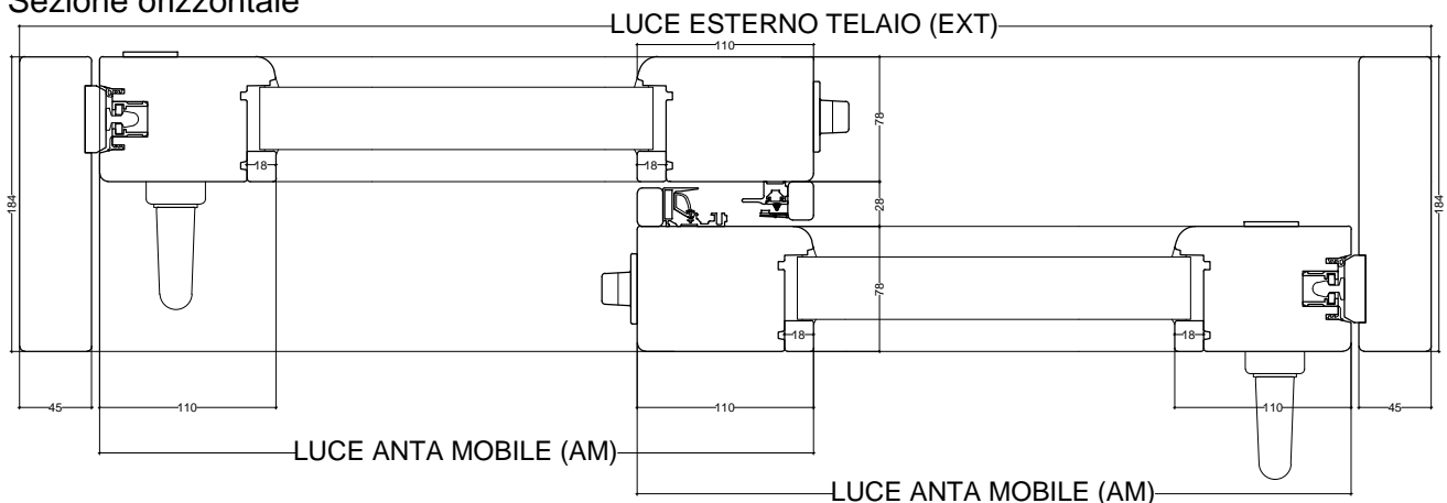
Sezione orizzontale
