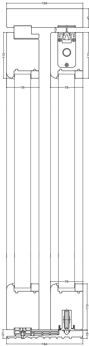
Sezione verticale
