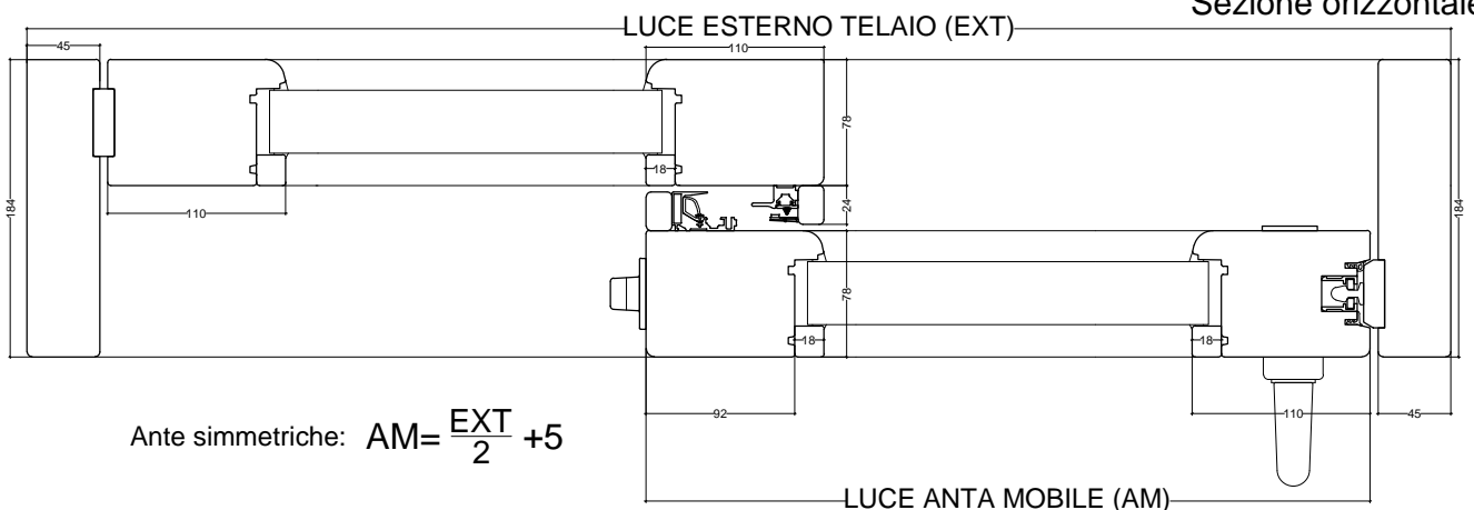
Sezione orizzontale
