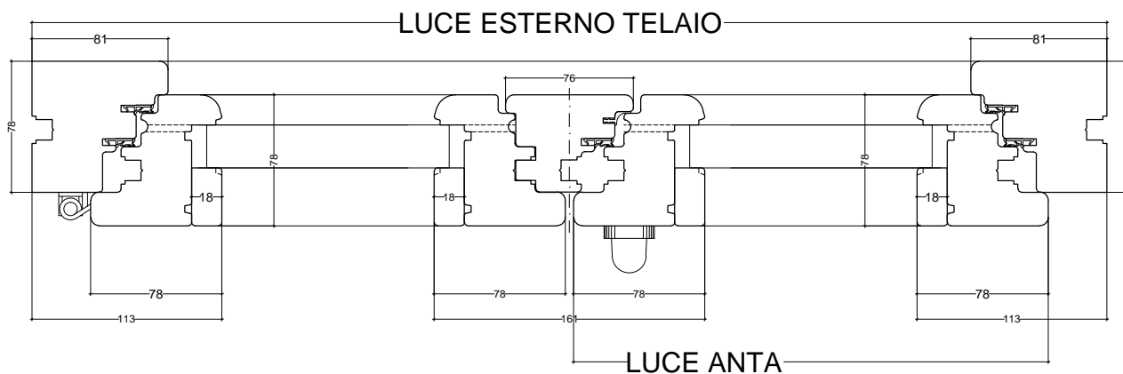
Sezione orizzontale
