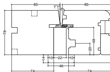
Sezione orizzontale E-F sotto le cerniere
