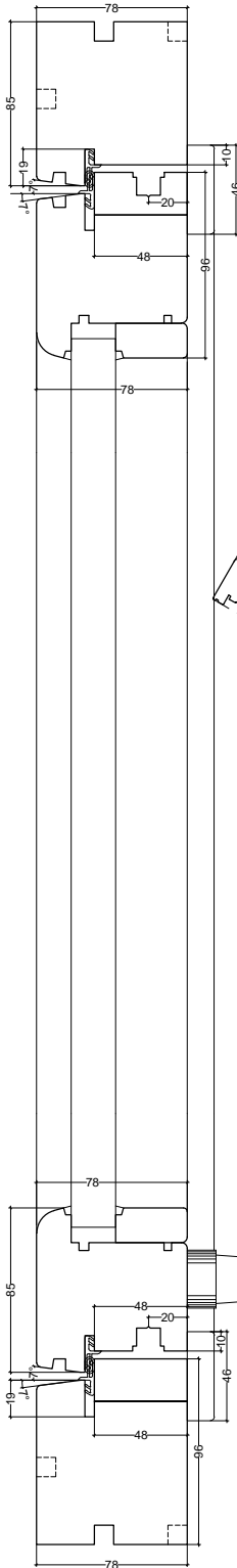
Sezione verticale A-B
