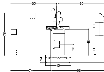
Sezione orizzontale C-D sopra le cerniere
